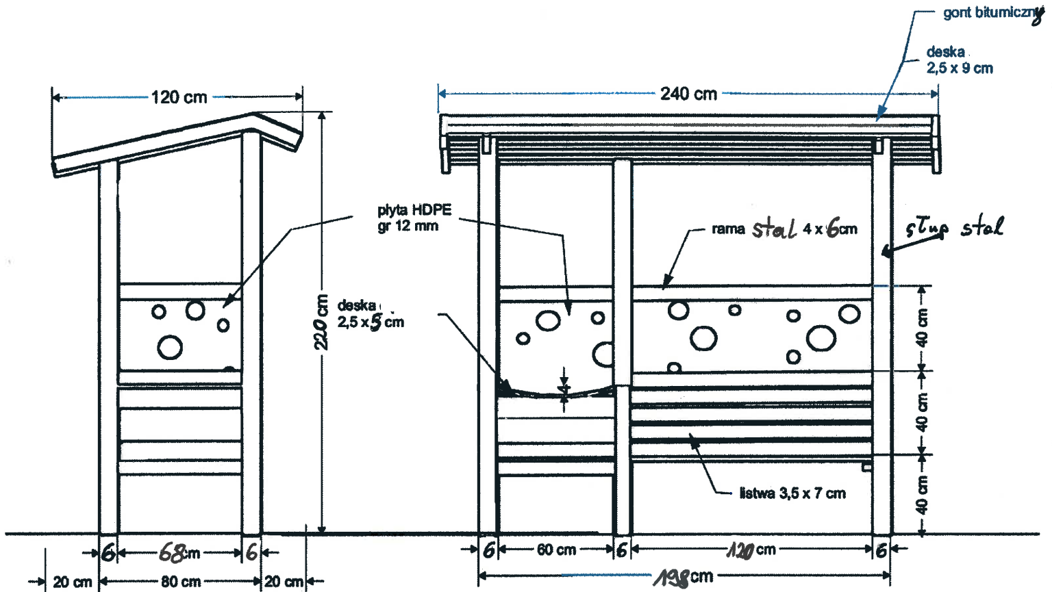
Rysunek techniczny - ławka dla matki z dzieckiem
